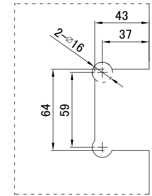
B詳細図 ヒンジガラス加工図 S=1/3
